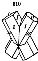
Staurolite.
